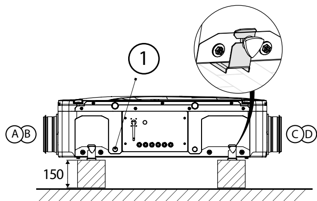
Abb. 2. Bodenmontage
