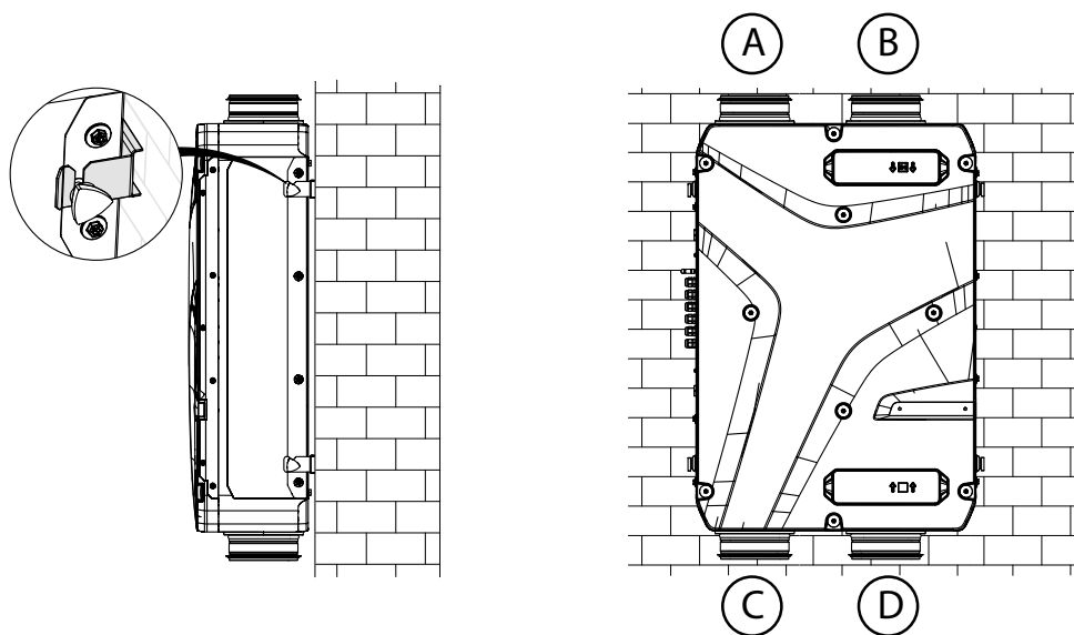
Abb. 5. Vertikale Wandmontage
