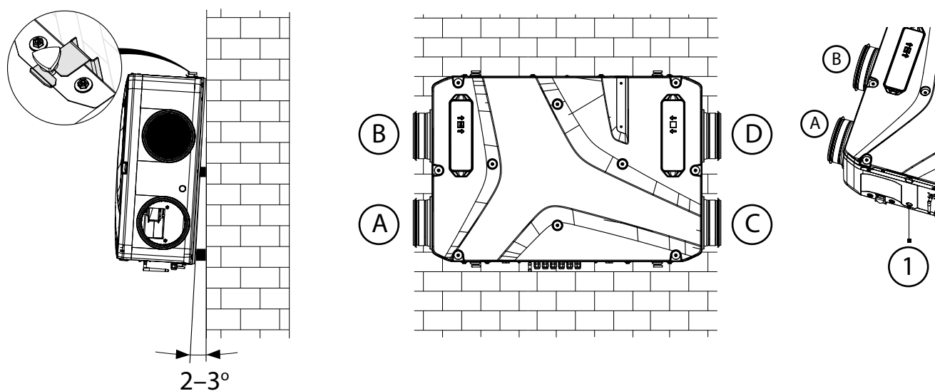
Abb. 4. Horizontale Wandmontage
