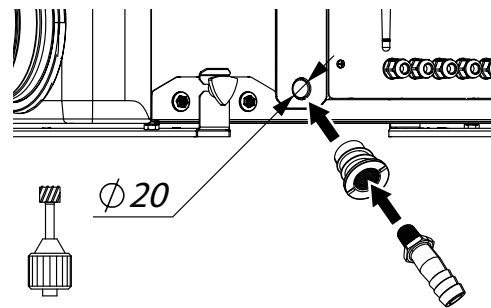
Montage des Ablaufstutzens bei der Montage der Anlage nach Abb. 2-4
