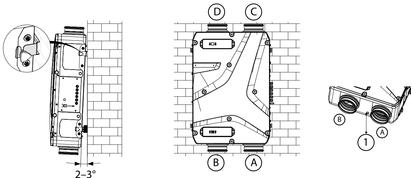
Abb. 3. Vertikale Wandmontage
