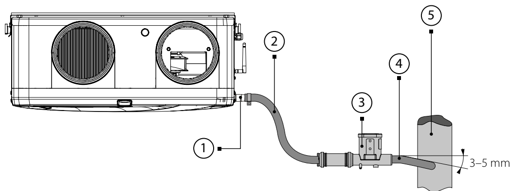
1: Ablaufstutzen, 2: Anschlussrohr, 3: Siphon, 4: Anschlussrohr, 5: Abwassersystem
