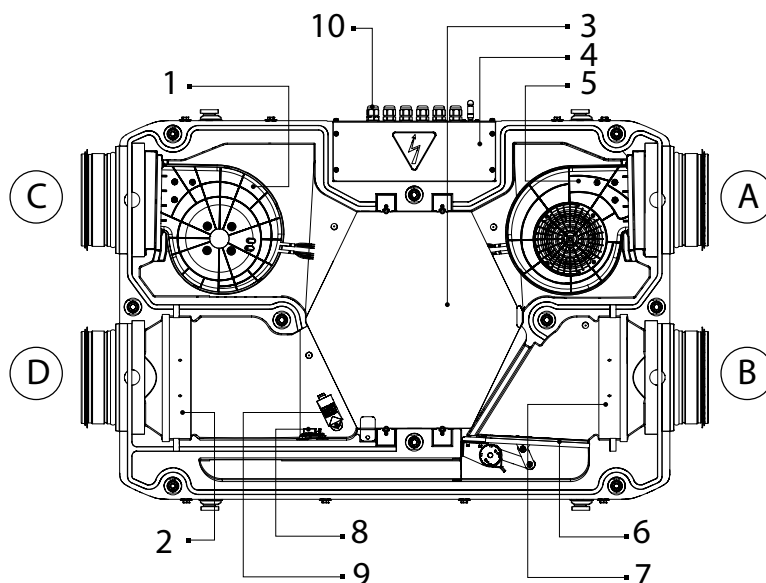
Ansicht bei abgenommener Wartungsblende
